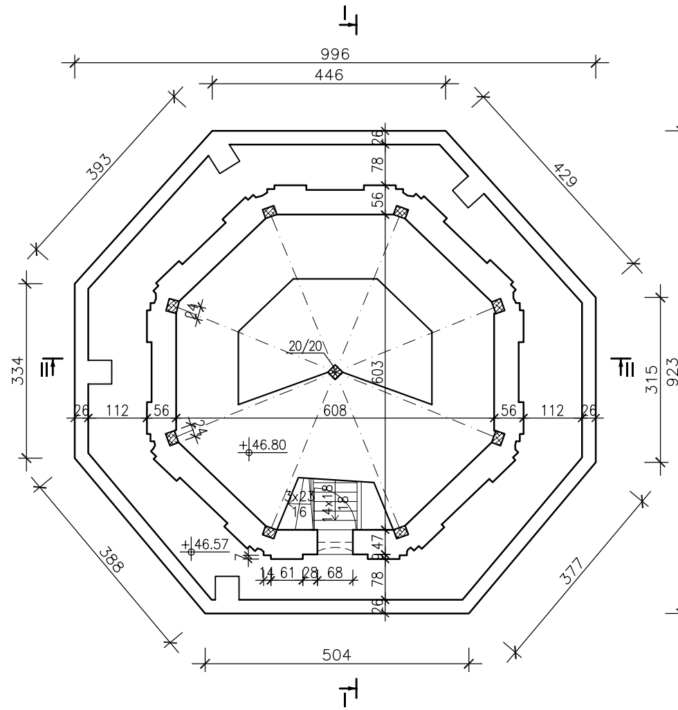
KONDYGNACJA XI
