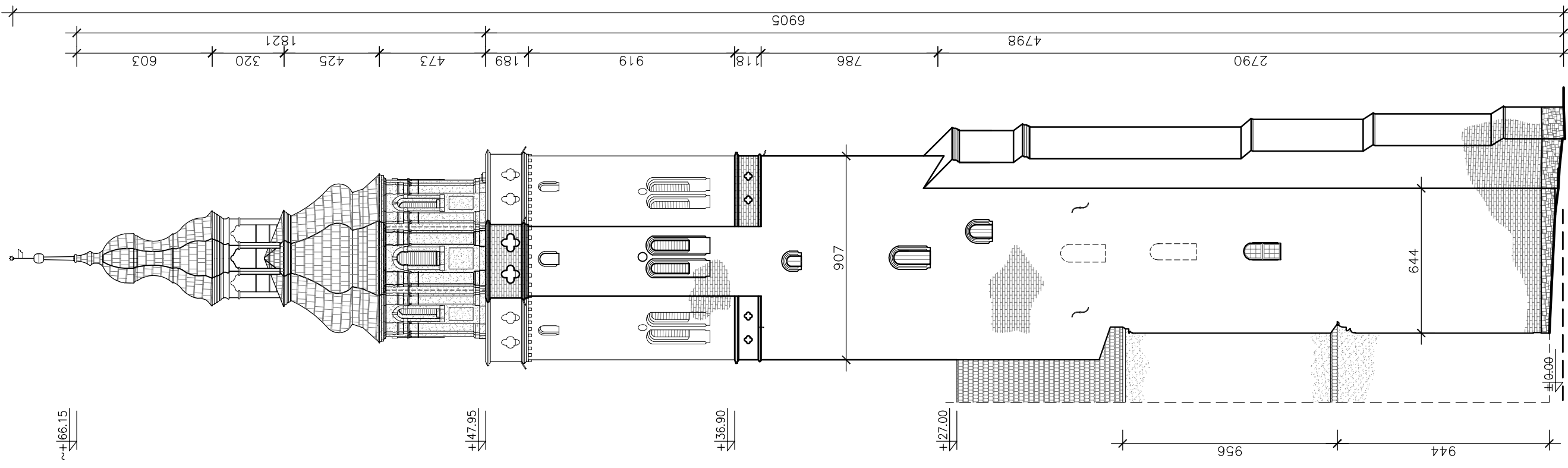
ELEWACJA PÓLNOCNA
