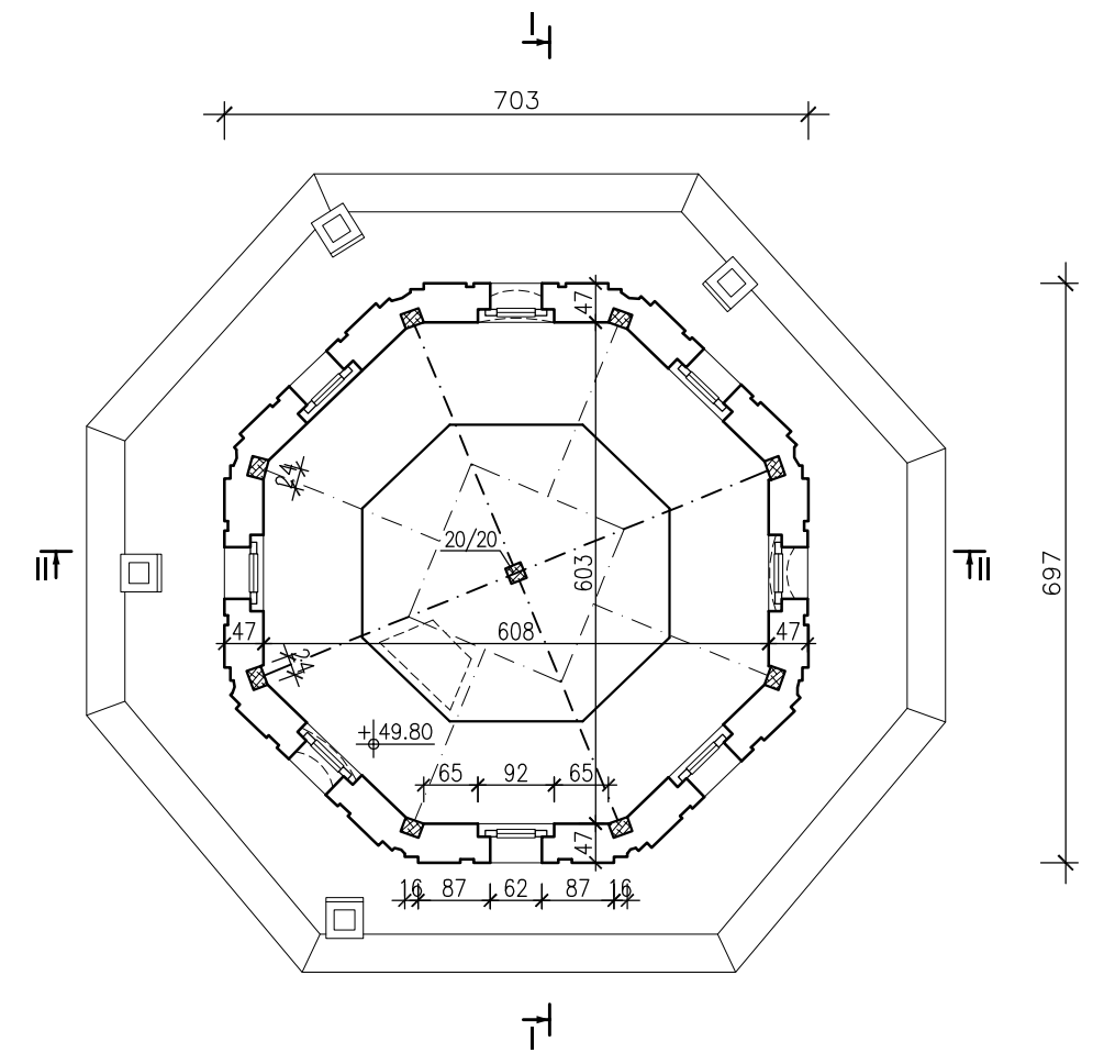
KONDYGNACJA XII
