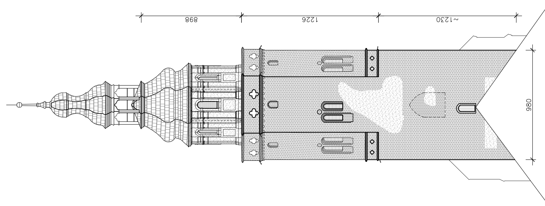
ELEWACJA WSCHODNIA
