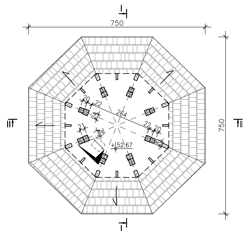
KONDYGNACJA XIII
