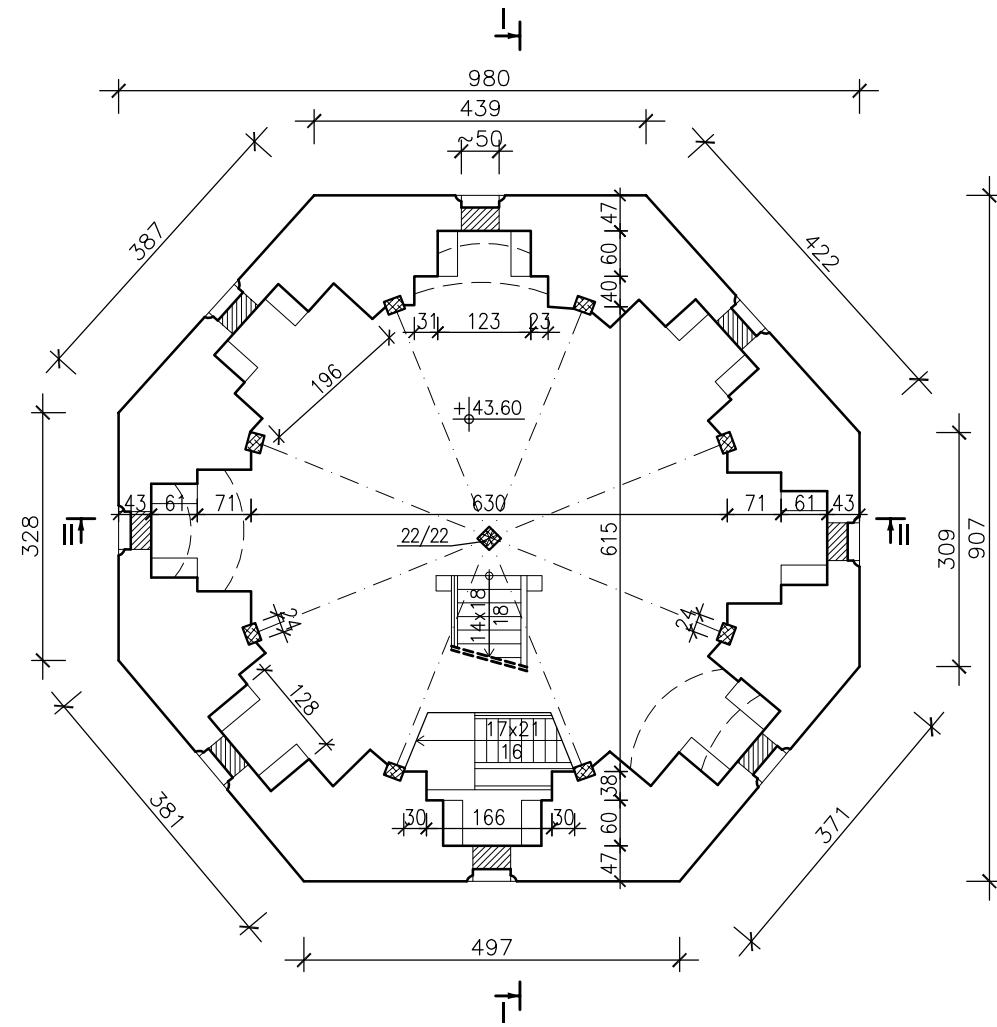
KONDYGNACJA X
