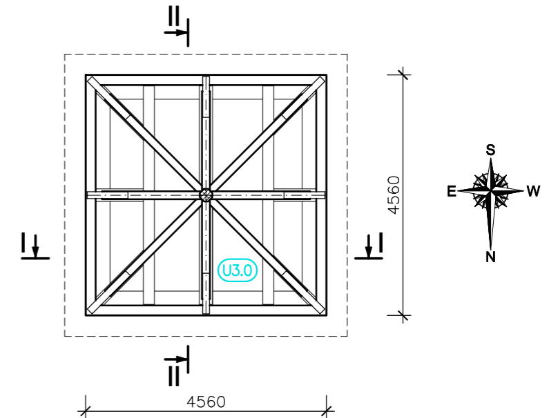
WIĘZ BA DACHOWA
